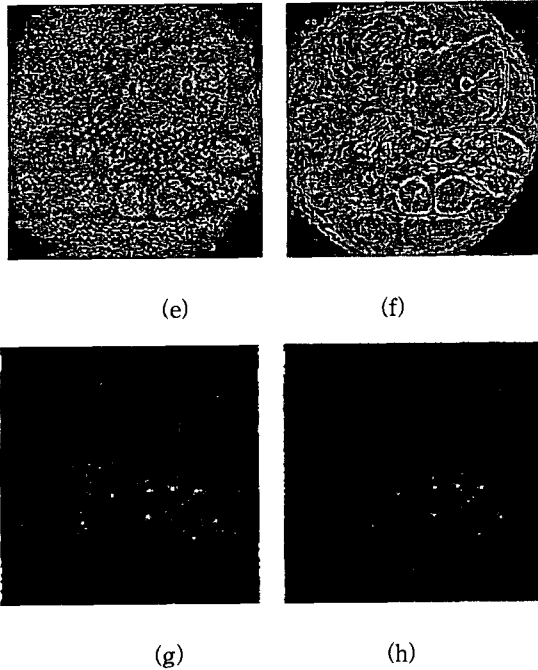
그림 3. 에지 검출
