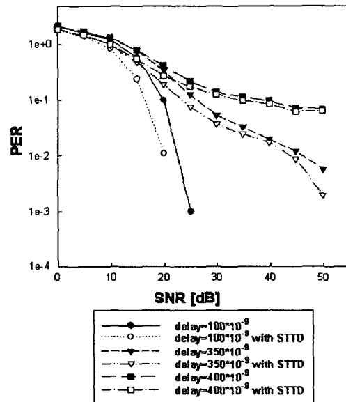
그림 6. 다중경로 페이딩 환경에서 STTD를 적용한 64QAM시스템의 성능 Fig. 6 Performance of 64QAM system with STTD in multipath fading environment
