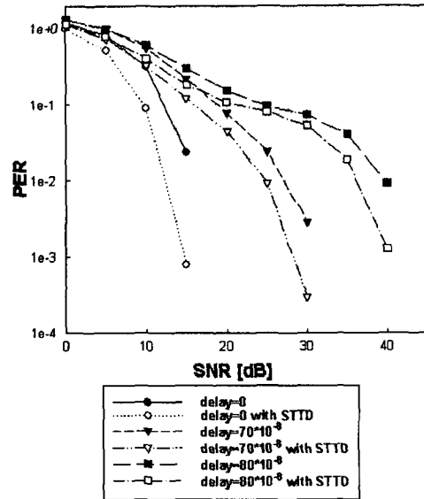
그림 5. 다중경로 페이딩 환경에서 STTD를 적용한 16QAM시스템의 성능 Fig. 5 Performance of 16QAM system with STTD in multipath fading environment
