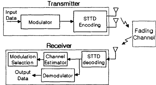
그림 2. STTD를 적용한 적응변조 시스템 모델 Fig 2. Adaptive modulation system model with STTD
