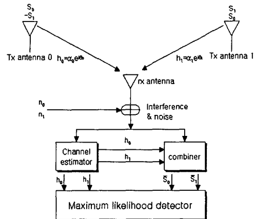
그림 3. 시공간 전송다이버시티 기법 Fig. 3 Space time transmit diversity scheme
