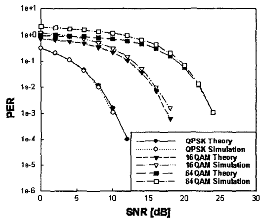
그림 4. AWGN 환경에서 각 변조방식에 따른 성능 Fig. 4 Performance according to modulation mode in AWGN environment
