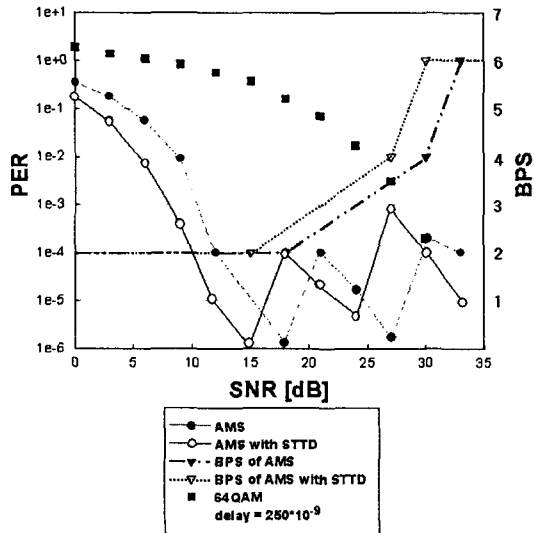
그림 9. 다중경로 페이딩 환경에서 적응변조 시스템의 성능 분석
