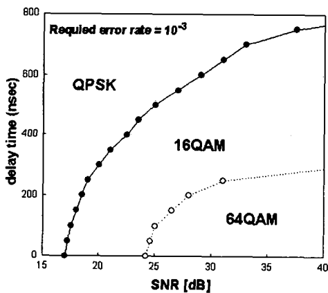
그림 7. 변조 모드 결정을 위한 기준 Fig. 7 Chart for selecting modulation scheme
