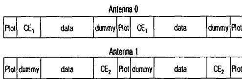
그림 1. 각 안테나의 프레임 구조 Fig 1. Frame structure of each antenna
