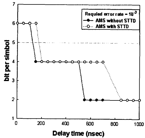
그림 8. 지연시간에 따른 적응변조 시스템의 전송용량 분석 (SNR=25dB)
