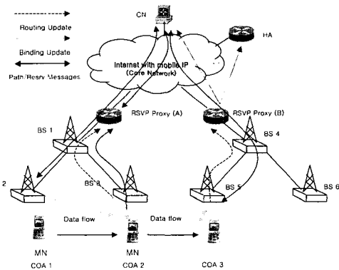
그림 3. Cellular IP와 RSVP 통합 모델
