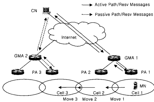
그림 2. HMRsVP의 예약 경로
