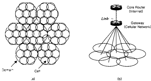
그림 7. 도메인 구성(a) 및 셀룰러 네트워크 토폴로지(b)
