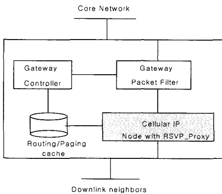
그림 4. 게이트웨이와 RSVP proxy 상호 운용
