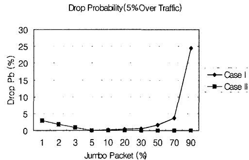
그림 6. 트래픽 폭주가 5% 초과 시 일반패킷 손실율 비교
