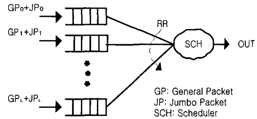
그림 1 점보패킷을 고려하지 않는 패킷 스케줄링
