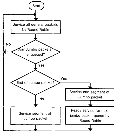
그림 3. 점보패킷 스케줄링 알고리즘
