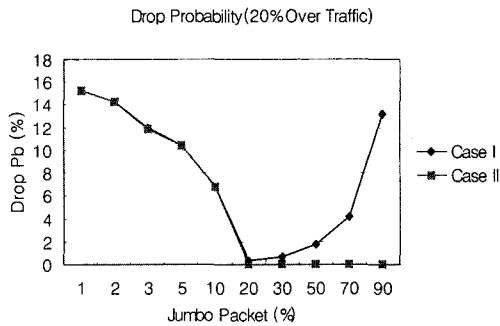
그림 7. 트래픽 폭주가 20% 초과 시 일반패킷 손실율 비교
