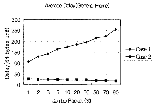
그림 5. 정보패킷 전달 시 일반패킷 전달 지연 비교
