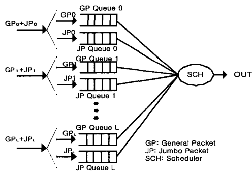
그림 4. 독립된 큐를 이용한 정보패킷 스케줄링
