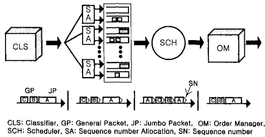
그림 2. 제안된 점보패킷 처리 블록도
