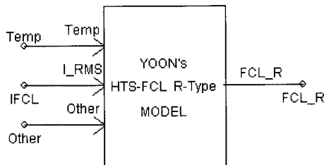
(a) 저항형 초전도한류기 EMTDC 모델 개요도 (a) EMTDC Model Layout of R-type HTS-FCL
