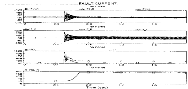
그림 6. 초전도한류기의 최종저항값 비선형 특성을 고려한 경우의 해석결과
