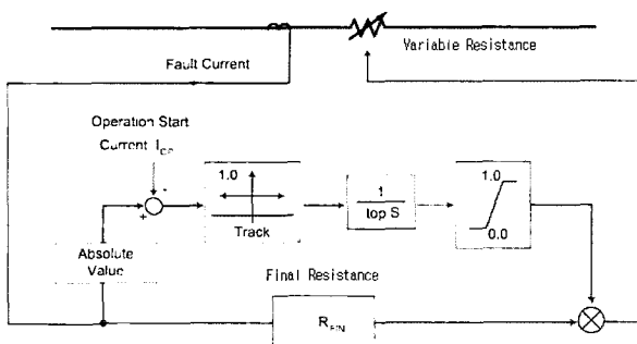
그림 1. 저항형 초전도한류기 대표모델 Fig. 1. Standard Model of R-type HTS-FCL
