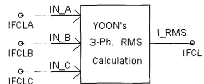
그림 2. 3상 전류 실효치 계산 알고리즘 Fig. 2. RMS Computation Algorithm for 3 Phase Current
