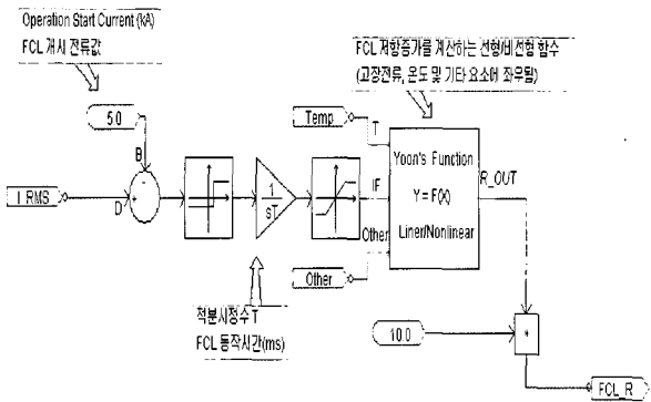
(b) 저항형 초전도한류기 EMTDC 모델 내용 (b) EMTDC Model Conternts of R-type HTS-FCL
