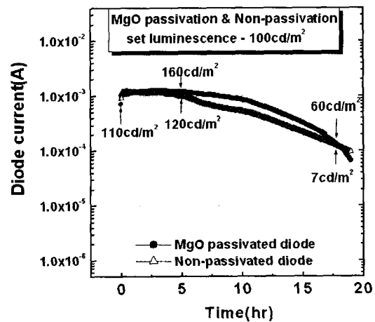
그림 4. 유기 EL 소자의 수명 및 휘도 특성. Fig. 4. Properties of the lifetime and luminescence from the OLED.
