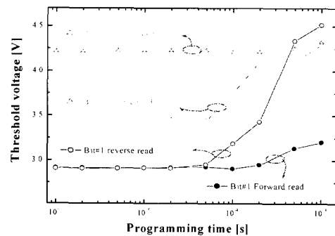
그림 6. 멀티 비트의 프로그램 특성. Fig. 6. The programming characteristics of multi-bit.
