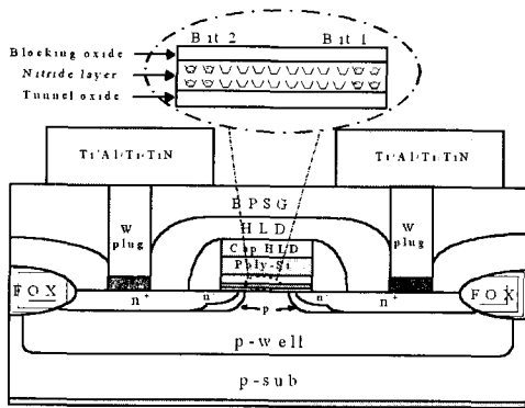
그림 1. SONOS형 멀티 비트 소자의 단면도. Fig. 1. The cross section of the SONOS type multi-bit device.
