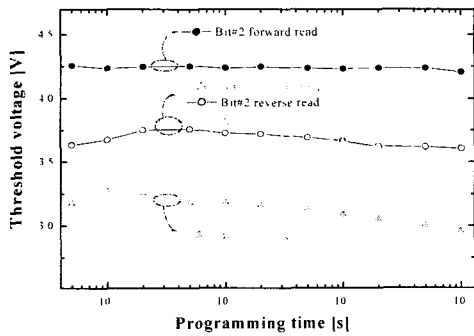
그림 7. 멀티 비트의 소거 특성.
