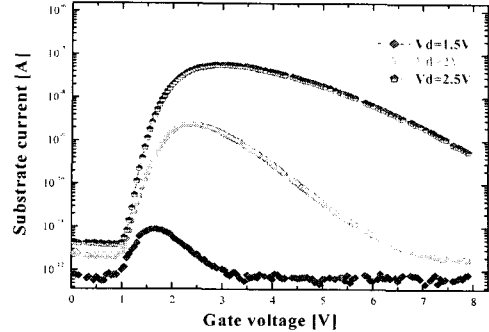
그림 2. SONOS형 멀티 비트 소자의 기판 전류 특성. Fig. 2. The substrate current of the SNOS type multi-bit device.
