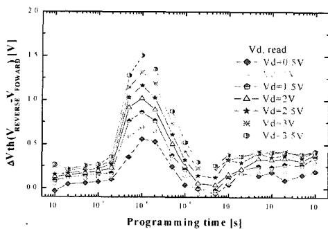
그림 5. 읽기 전압변화에 따른 멀티 비트 프로그램 특성. Fig. 5. The programming characteristics of multi-bit depending upon the reverse read voltage.
