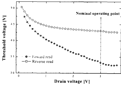
그림 4. 멀티비트의 문턱전압 대 읽기 동작을 위한 드레인전압. Fig. 4. Threshold voltage of multi-bit of the cell vs. the drain voltage for read operating.
