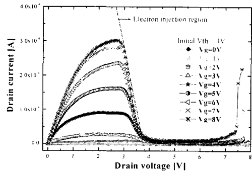
그림 3. SONOS형 멀티 비트 소자의 원-샷 프로그래밍 곡선. Fig. 3. The one-shot programming curve of the SONOS type multi-bit device.
