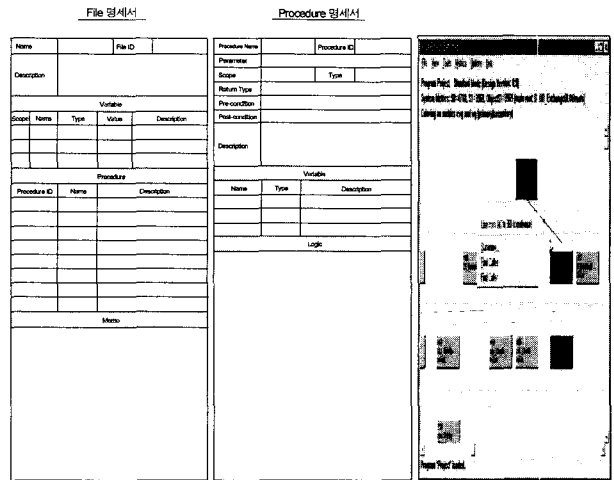
(그림 9) File, Module Description Template, Structure Chart(McCave의 Battlemap)
