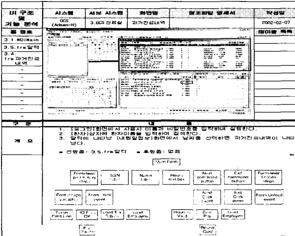
(그림 8) UI 기능, 구조 명세서
