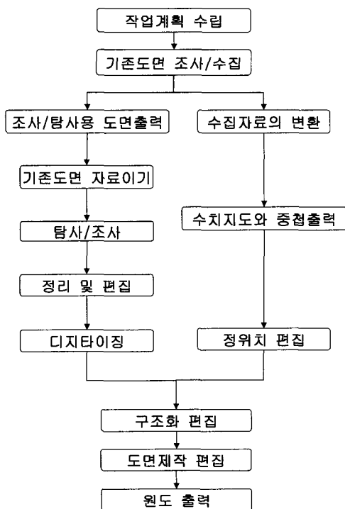
그림 4. 표준화된 지하시설물 조사/탐사 및 입력 공정
