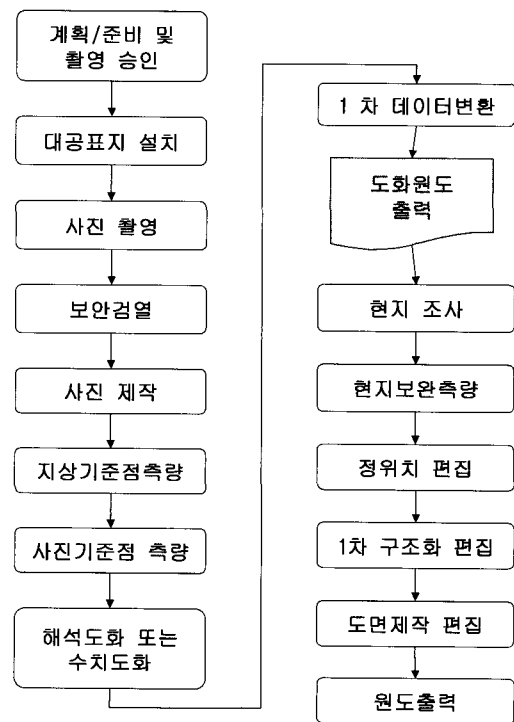
그림 2. 표준화된 수치지도 신규제작 공정
