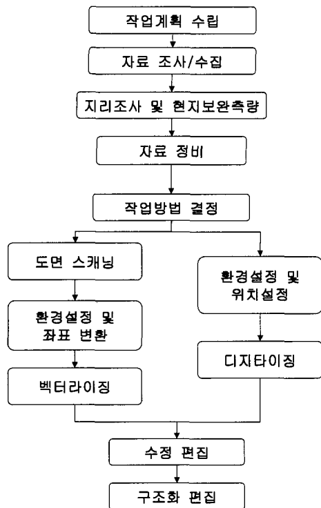
그림 3. 표준화된 기존도면입력 공정
