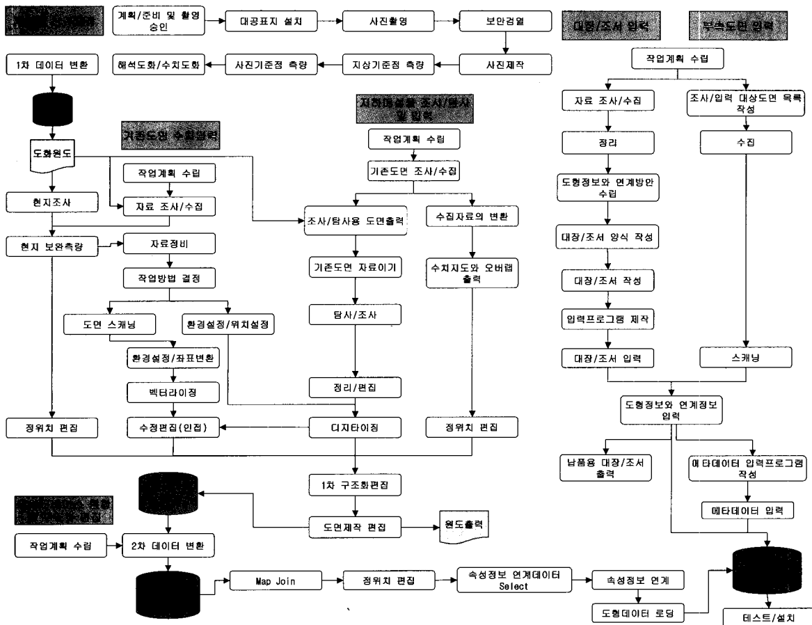
그림 1. 표준화된 공간데이터베이스 구축공정
