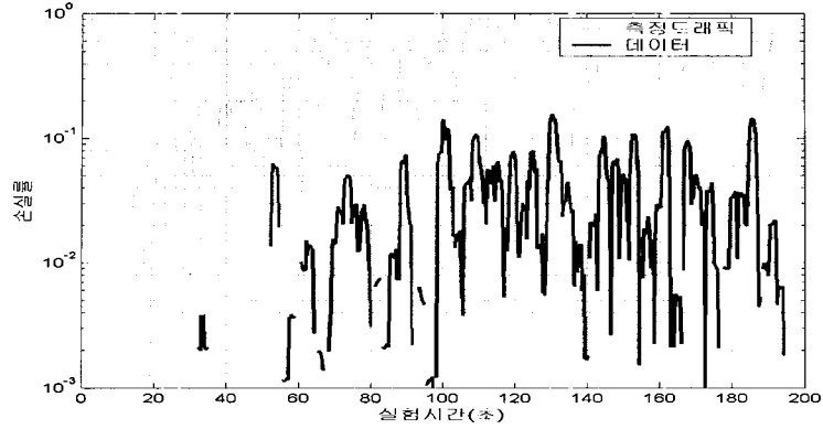
그림 9. 목표 손실률이 0.1일 때, 데이터 트래픽과 추정 트래픽의 손실률 Fig. 9. Loss rate of both data and probe traffic when the target loss rate = 0.1.
