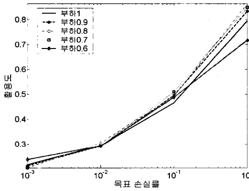
그림 10. 목표 손실률의 증가에 따른 활용도 곡선 Fig. 10. Utilization v.s. target loss rate
