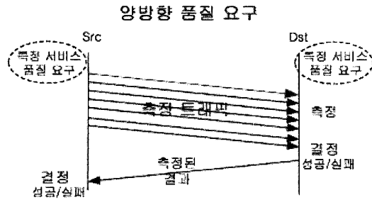
그림 3. 송신자 수신자 모두 QoS를 요구할 때 Fig. 3. When sender and receiver both demand their QoS
