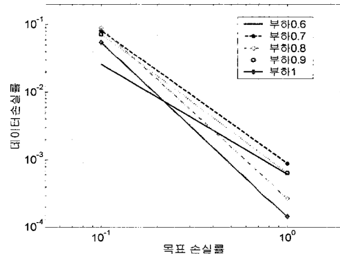
그림 11. 목표 손실률의 증가에 따른 데이터트래픽 손실률 Fig. 11. data loss rate v.s. target loss rate.
