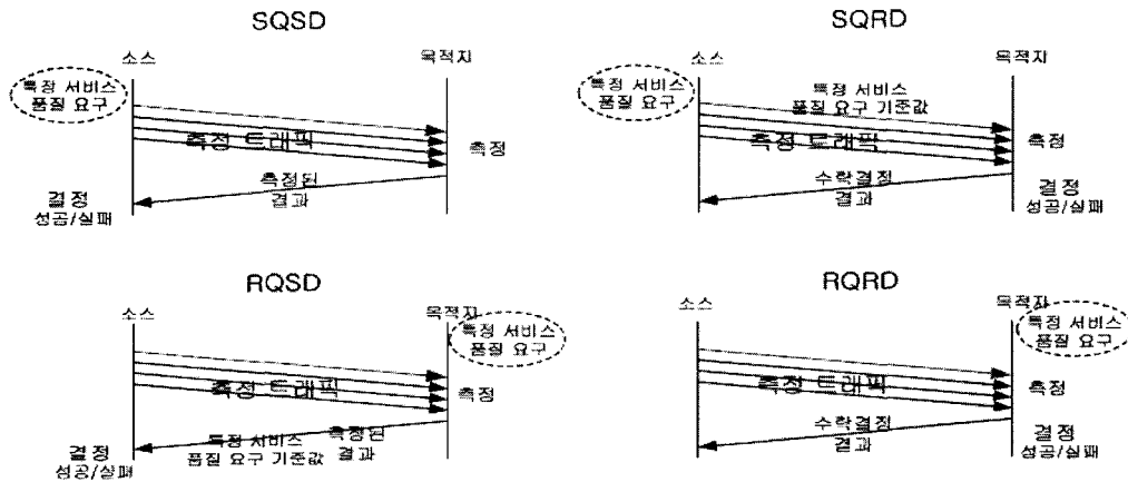
그림 2. QoS 요구 위치와 수락여부 결정 위치에 따른 EMBAC 기법들의 종류 Fig. 2. Types of EMBAC schemes according to where to demand QoS and decide admission.
