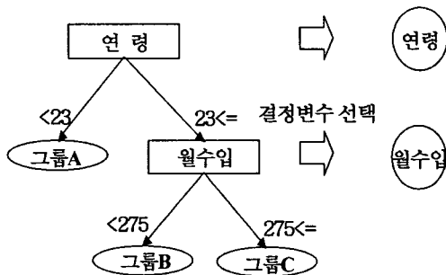
<그림 1> 결정변수의 선택과정
