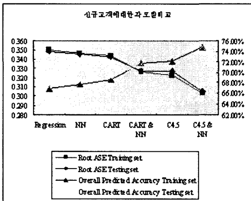
<그림 10> 신규고객에 대한 각 모델비교
