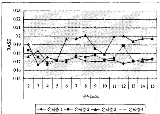
<그림 8> 은닉노드와 은닉층의 변화 (기존고객의 평가집합)
