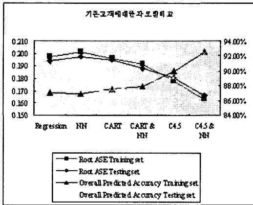
<그림 9> 기존고객에 대한 각 모델비교
