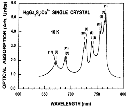
그림 5. HgGa 2 S 4 :Co 2+ 단결정의 불순물 스펙트럼(10 K).
