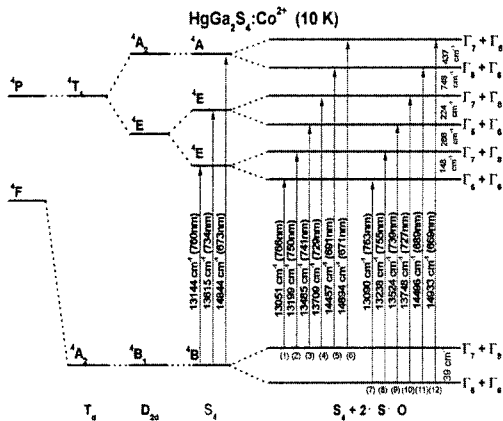
그림 6. HgGa 2 S 4 :Co 2+ 단결정에서 Co 2+ (S 4 ) 이온의 에너지 준위 분리와 전자전이 모형(10 K).
