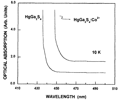
그림 1. \text{HgGa}_2\text{S}_4 및 \text{HgGa}_2\text{S}_4:\text{Co}^{2+} 단결정의 기초 흡수단 영역에서 광흡수 특성.
