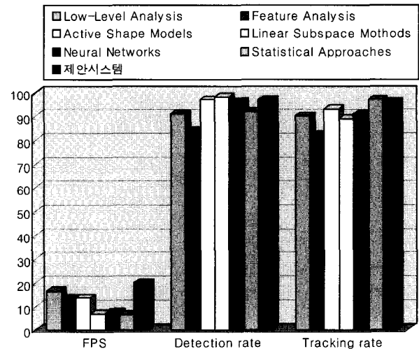
(그림 16) 시스템 성능 비교
