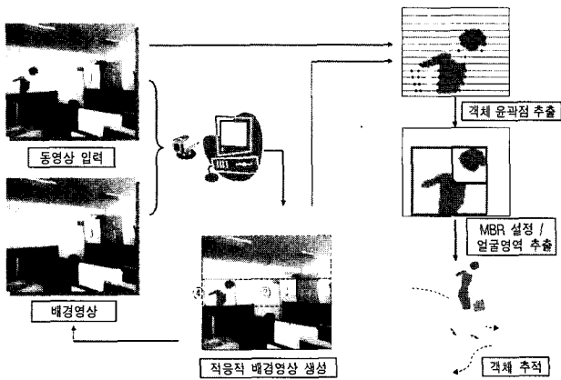
(그림 1) 시스템 처리 흐름도
