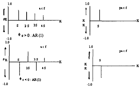
<그림 2> 안정적 계절 AR(1)과 MA(1)의 이론적 ACF와 PACF
