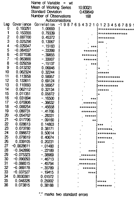
<그림 6> 원시계열의 자기상관함수 ACF
