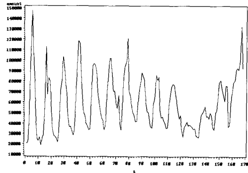
<그림 4> 원시계열 불규칙요인 변동추이
