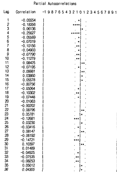
<그림 11> 추정된 모형에의한 잔차분석 : PACF
