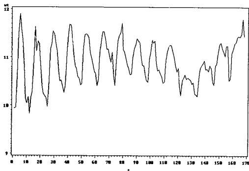
<그림 5> 원시계열 대수변환그래프
