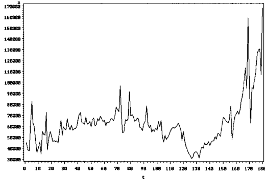
〈그림 12〉 최종계절 변동 조정시계열 그래프
