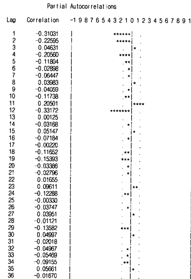
<그림 9> 시계열의 1차 차분후의 PACF
