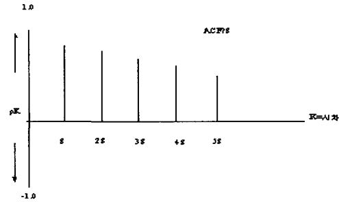
<그림 3> 불안정적 평균을 지니는 계절적 계열과정의 ACF
