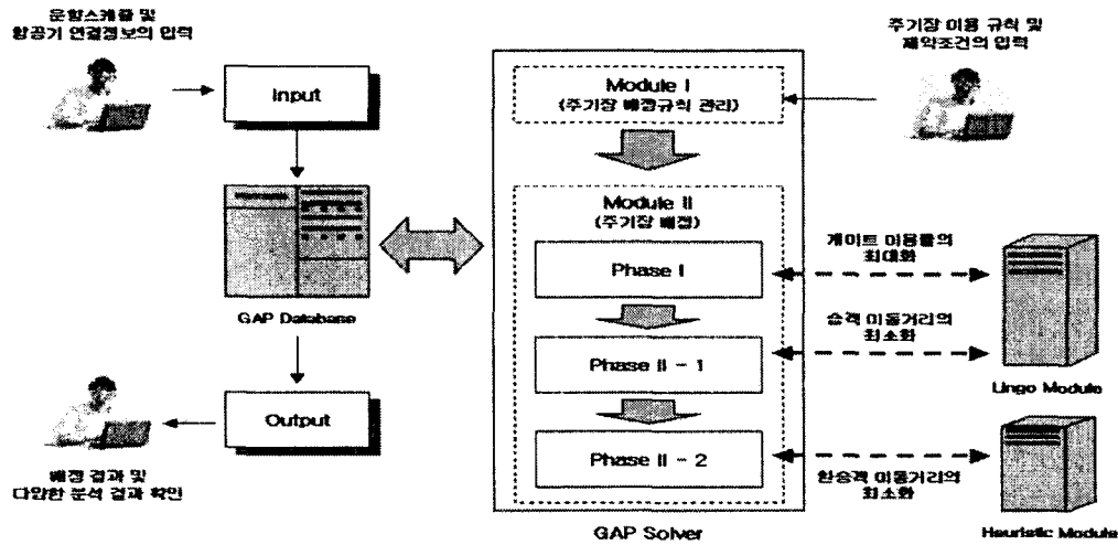
<그림 2> 의사결정지원시스템 구성도
