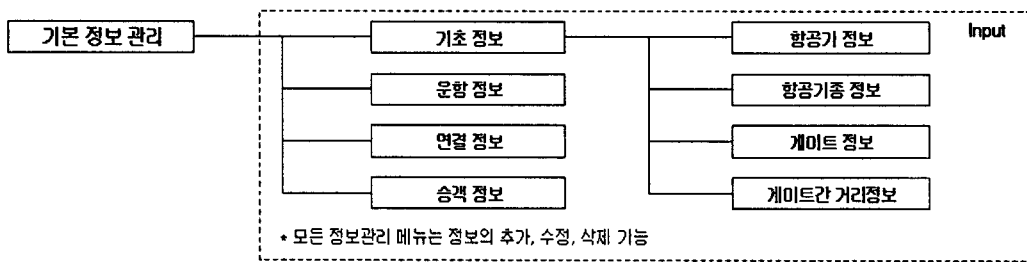
<그림 4> 기초정보 관리의 메뉴 구성도
