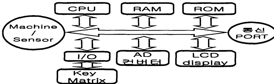
<그림 4> 정보처리 HARDWARE 구성도
