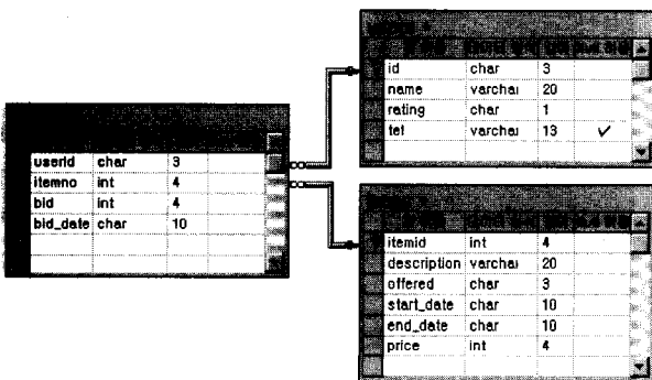
(그림 3) 관계형 데이터베이스 스키마
