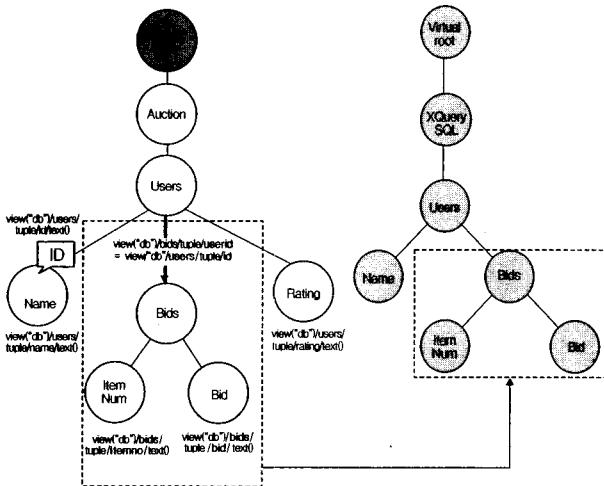
(그림 11) 질의 트리 생성 과정 2
