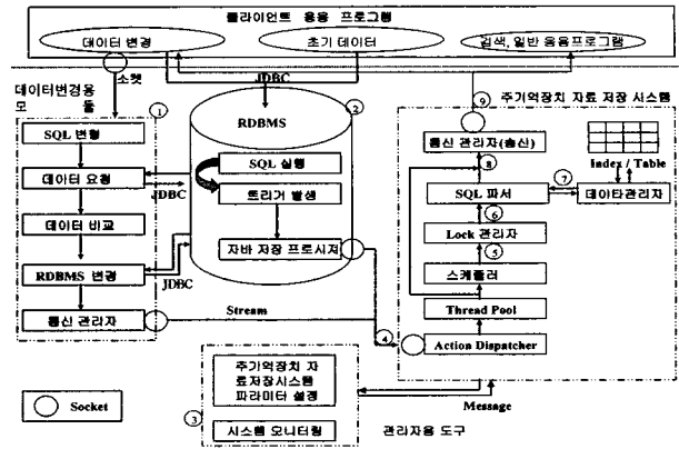
(그림 4) 프로그램 처리 절차
