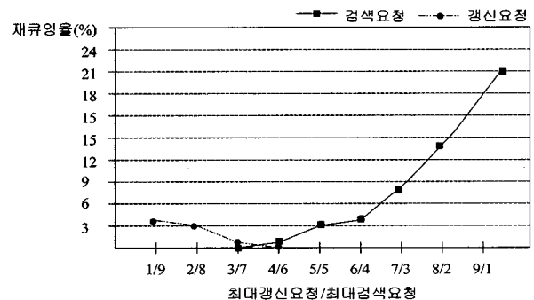
(그림 8) 갱신/검색 요청에 따른 재큐잉률
