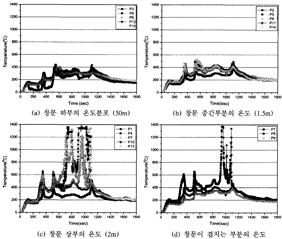
그림 5. 창문 주위의 온도분포도.
