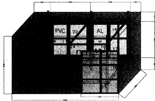
그림 3. 건물 내부의 온도측정 위치.
