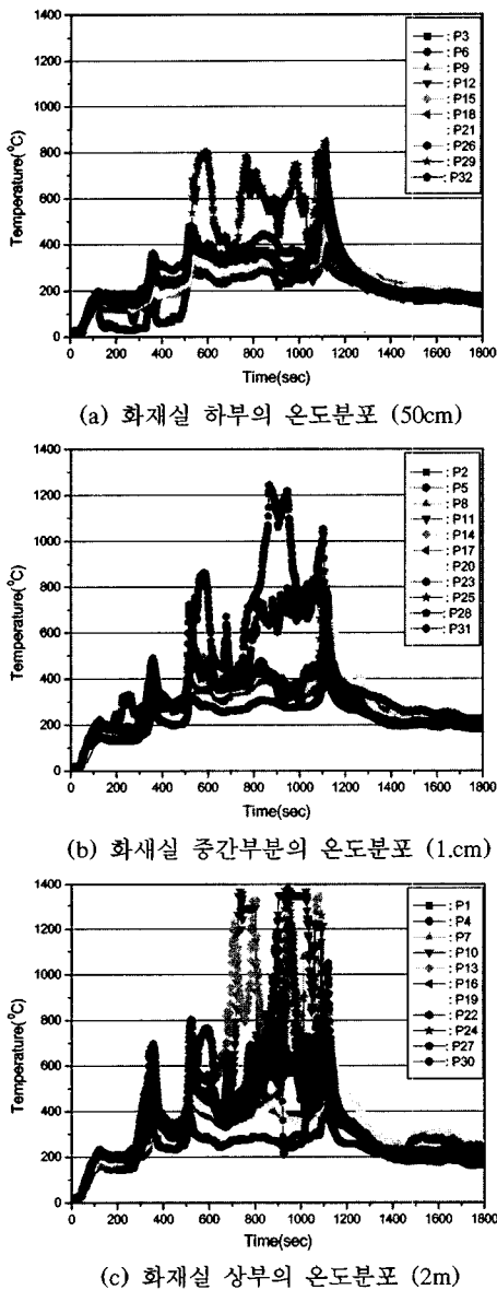
그림 4. 건물 내부의 온도분포도.
