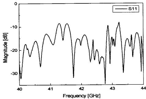
그림 6. 슬롯 배열 안테나의 반사계수(측정치) Fig. 6. Measured results of return loss.
