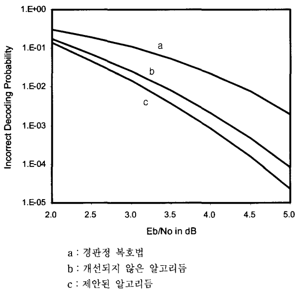
(그림 1) (63, 36) BCH 부호에 대한 복호 에러 확률
