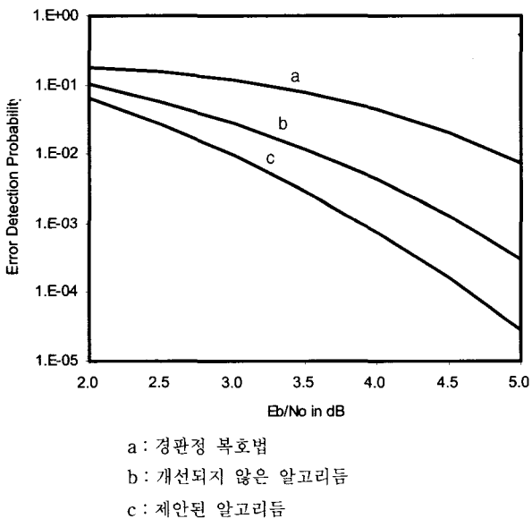
(그림 2) (63, 36) BCH 부호에 대한 에러 검출 확률
