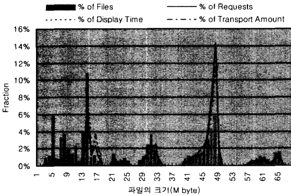
(그림 4) B서버의 파일 크기에 따른 요구 분포
