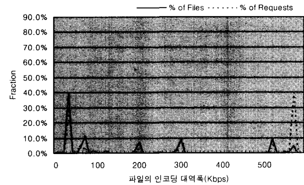
(그림 8) C서버의 파일의 인코딩 대역폭에 따른 요구 분포
