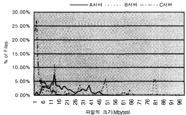
(그림 2) 각 서버별 연속미디어 파일의 크기 분포
