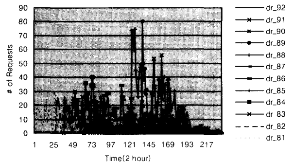
(그림 15) 주 5회 생성되는 시리즈 연속미디어 파일의 요구수 분포
