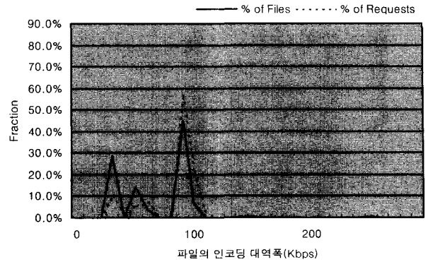
(그림 6) A서버의 파일의 인코딩 대역폭에 따른 요구 분포
