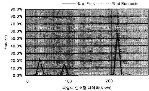
(그림 7) B서버의 파일의 인코딩 대역폭에 따른 요구 분포
