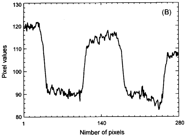
그림 4. (A)는 11-MUA의 표면 플라즈몬 이미지이다. 원래 지름 \phi=300\ \mu\text{m} 인 원형의 각 채널은 반사광의 굴절로 인하여 약간 변형된 타원형으로 보인다. (B)는 (A)의 네모로 표시된 부분의 종방향으로 20 화소 값을 평균한 Line profile이다. 이로부터 단분자막의 두께를 정량적으로 보정하면 임의의 시료의 두께 변화를 알 수 있다. (B)에서 오른쪽 채널의 밑면이 아래로 치우친 것은 얻어진 전체 이미지에서의 음영에 의한 것이다.
