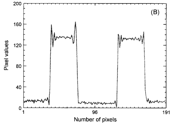
그림 3. (A) 2 nm의 크롬(Cr)과 45 nm의 금(Au), 그리고 약 920 nm 두께의 Photoresist(AZ5214E)가 코팅된 500 \mu\text{m} \times 500 \mu\text{m} 크기의 채널이 패터닝 된 센서 칩의 표면 플라즈몬 이미지. 네 개의 채널만 나타내었음. (B) (A)에서 직선으로 표시된 부분의 Line profile을 화소 값으로 나타낸 그림. 값으로 볼 때 PR이 코팅된 채널 부분이 바탕 면인 금 표면에 비해 100이상의 차이를 보인다.
