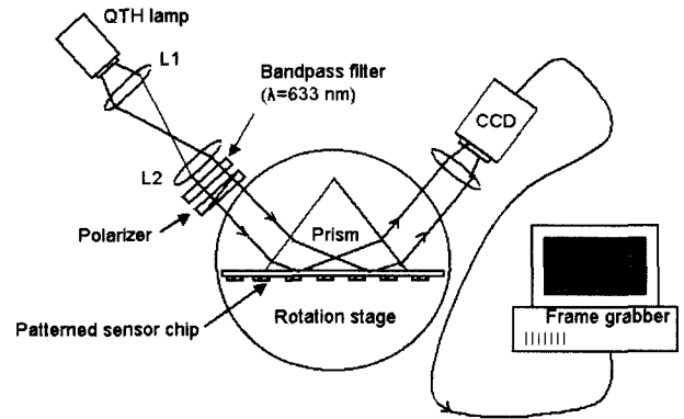
그림 1. 표면 플라즈몬 이미징 시스템의 개요도: 텅스텐-할로젠 램프(QTH lamp)에서 나온 빛은 렌즈(L1, L2)를 거쳐 평행광이 되고, 단색광을 얻기 위한 대역통과 필터(Narrow band-pass filter, λ 0 =633 nm, Δλ=1 nm)와 표면 플라즈몬의 공명 조건(TM-mode)을 만족 만족시키기 위한 편광기를 거쳐 지름 약 7mm의 평행광으로 프리즘에 입사된다. 단분자막이 패터닝 된 커버 글라스, 즉 센서 칩은 Index matching oil을 이용하여 삼각 프리즘에 부착된다. 그리고 센서 칩을 포함한 프리즘 커플러는 전기적으로 제어되는 θ-2θ Goniometer의 중심에 위치하고, 컴퓨터에 의해 제어되는 입사광의 각도의 변화에 따른 반사광은 1/3"의 CCD 칩이 장착된 768(H)×494(V)의 화소를 갖는 범용 CCD 카메라와 PC 내부에 장착된 Frame grabber에 의해 디지털화 되어 그림 파일로 저장 된다.
