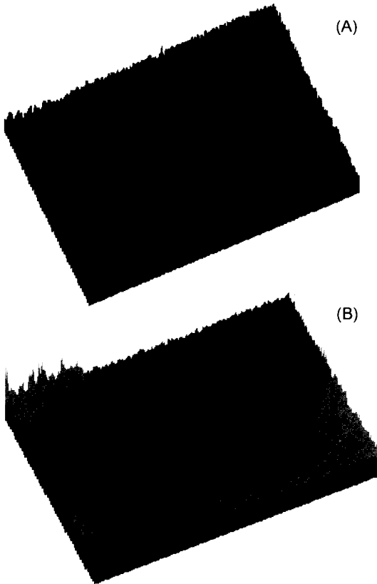
그림 6. 11-Mercaptoundecanol(11-MUOH) 단분자막에 대한 Surface plot: 실험적으로 구한 두께 변화에 대한 공명각의 변화는 약 1.31°인 11-MUA에 비해서 11-MUOH인 경우 0.068°로 11-MUA의 약 5% 정도로, 이루어진 막의 두께도 그에 따라 11-MUA의 경우 보다 훨씬 작다. 그리고 그림 5의 경우와 반대로 이 그림의 사각형 패턴은 일반적인 크롬 마스크를 이용하였기 때문에 사각형 패턴 부분에 11-MUOH 단분자막이 성막되어 있고 나머지 부분이 금 표면이므로 그에 따라 얻어진 영상의 요철이 그림 5와 비교해서 반대가 되었다. 즉 (A)에서의 어두운 부분이 금 표면에서의 플라즈몬 공명에 의한 흡수 조건에 상응하고, 밝은 부분, 즉 사각형 패턴이 11-MUOH 단분자막을 나타낸다.
