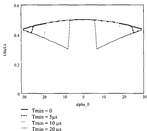
Fig. 17. Error of phase output voltage ( T_p=100\mu s ).
