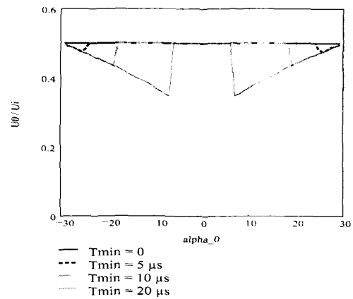
Fig. 15. Amplitude error of output voltage ( T_P=100\mu s ).
