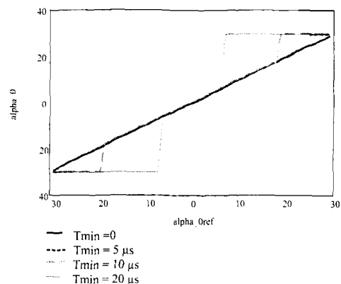
Fig. 16. Phase angle error of output voltage ( T_P=100\mu s ).
