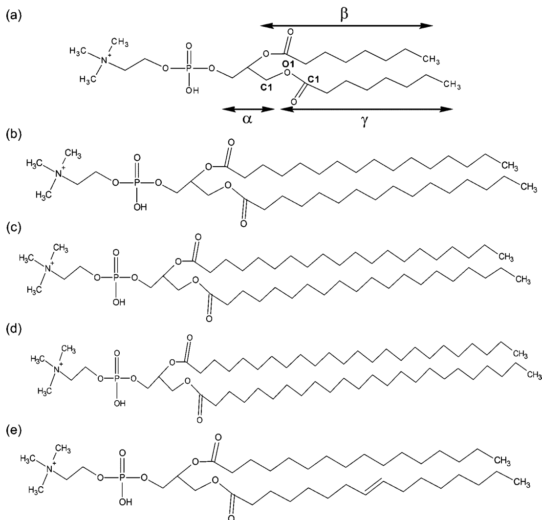
Figure 1. The chemical structure of (a) DOPC(C8), (b) DPPC(C16), (c) DAPC(C20), (d) DLPC(C24), (e) POPC.
