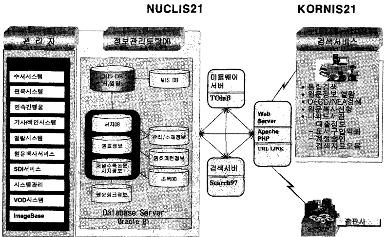
(그림 1) 시스템 구성도
