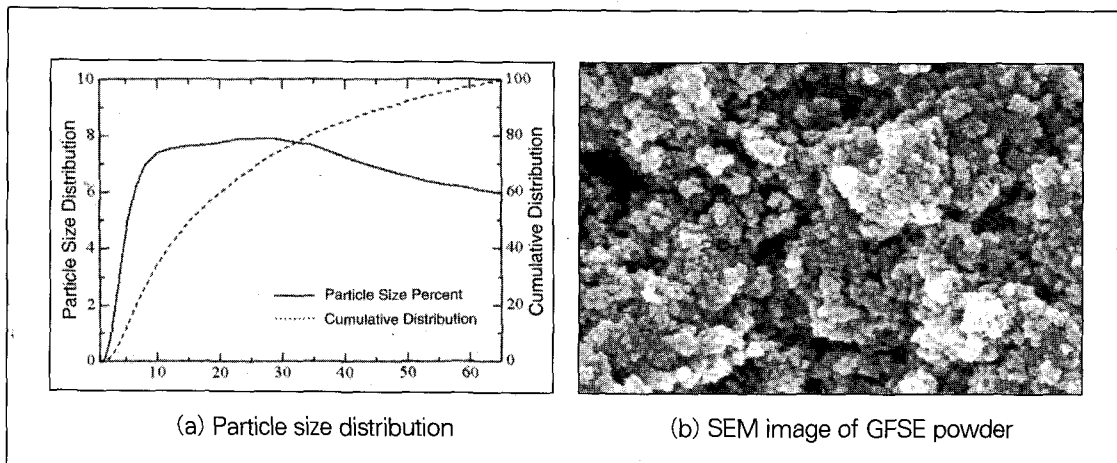
(사진 2) 기능성 첨가제(GFSE)의 입도 분포 곡선과 전자현미경(SEM)
