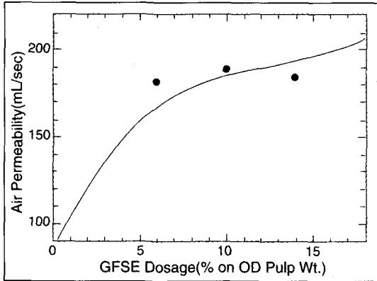
(그림 3) 기능성 첨가제 처리된 포장 원지 투기도 변화
