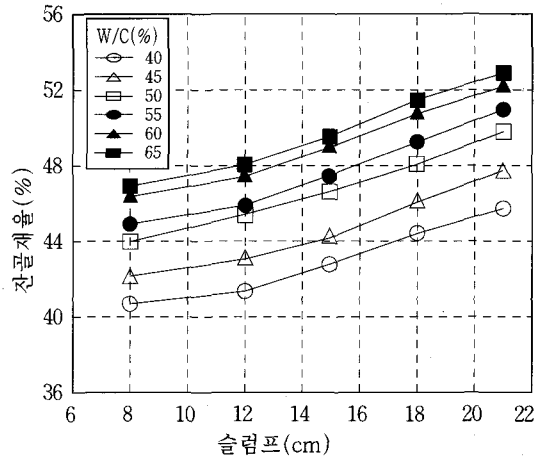
〈그림-3〉 보통 콘크리트의 잔골재율(부순돌 20mm)
