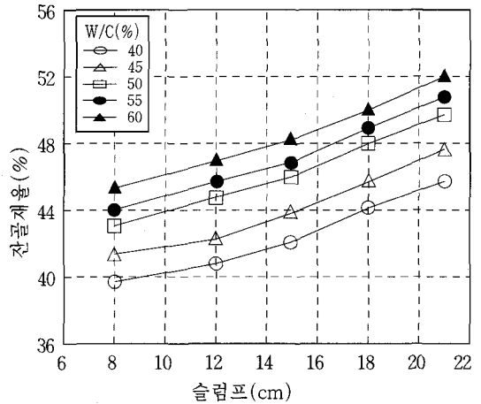
〈그림-5〉 경량 콘크리트 2종의 잔골재율
