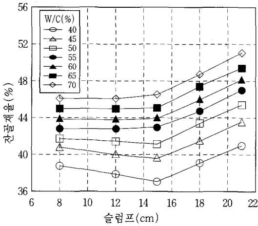
〈그림-2〉 보통 콘크리트의 잔골재율(강자갈 25mm)
