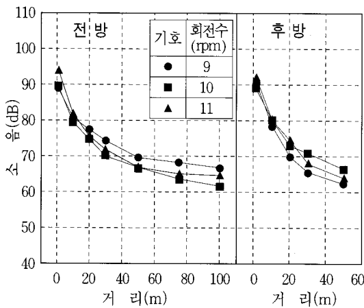
〈그림-9〉 거리에 따른 소음의 변화
