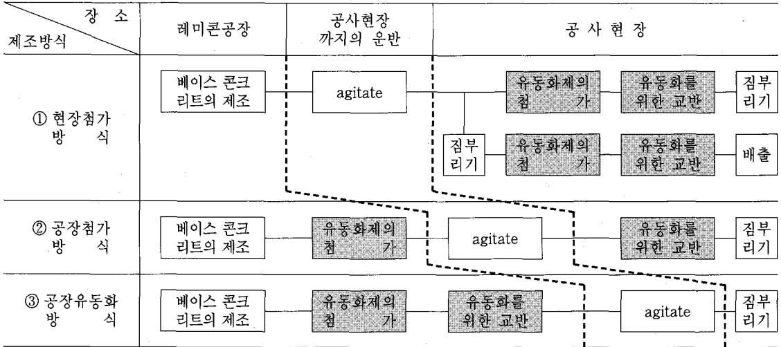
〈표-1〉 유동화 콘크리트의 제조 방법
