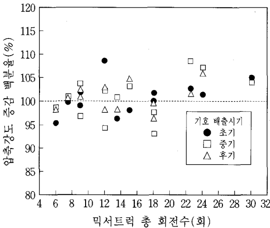
〈그림-7〉 에지테이터 트럭 총 회전수와 공기감소량
