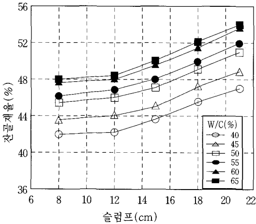
〈그림-4〉 경량 콘크리트 1종의 잔골재율
