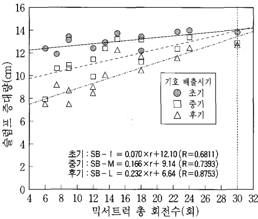
〈그림-6〉 에지테이터 트럭 총 회전수와 슬럼프 증대량
