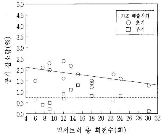
〈그림-8〉 에지테이터 트럭 총 회전수와 압축강도 증감백분율
