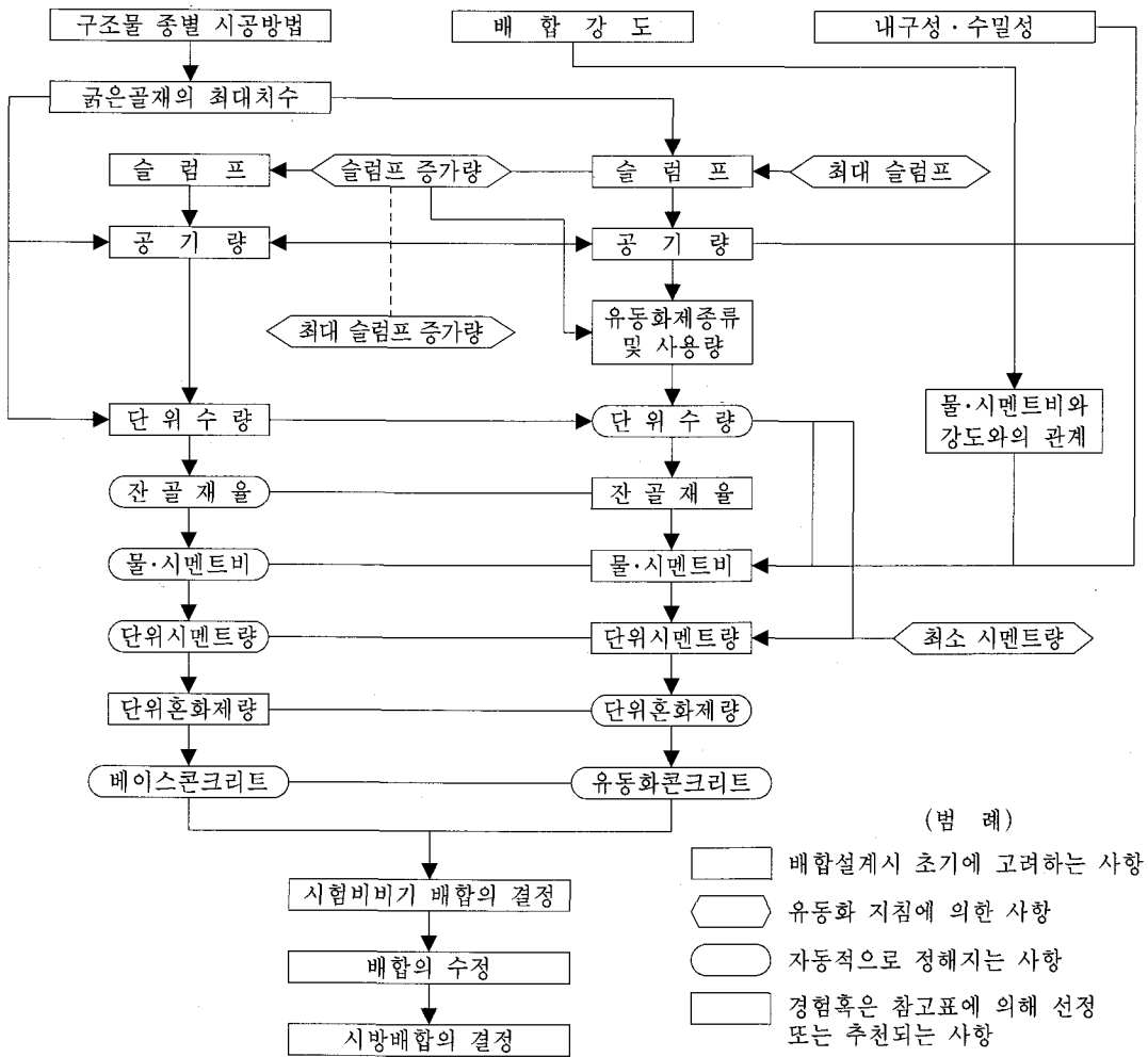
〈그림-1〉 유동화 콘크리트의 배합설계 흐름도
