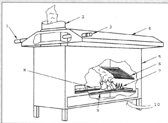
그림2. 바닥재 화재시험장치 구성도
