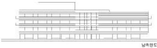
남측면도
