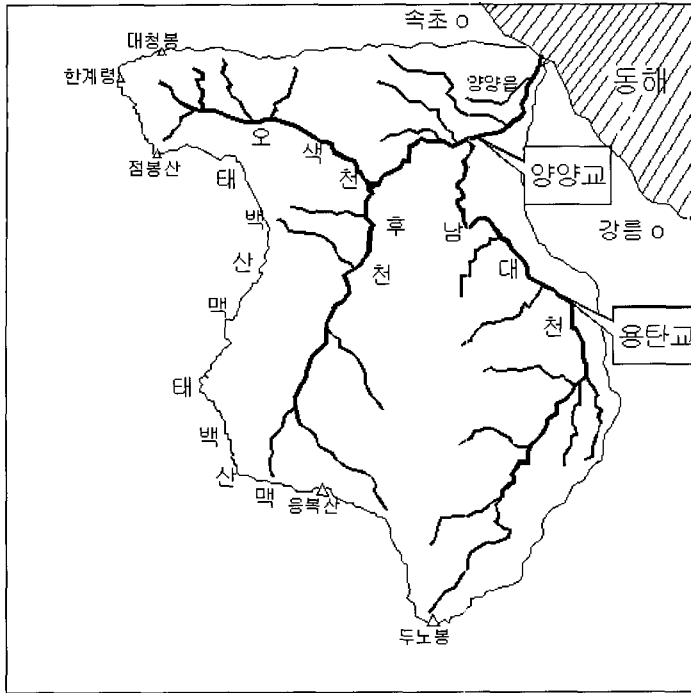
그림 1. 양양 남대천 유역도
