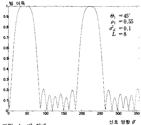
그림 4. 빔 형태
