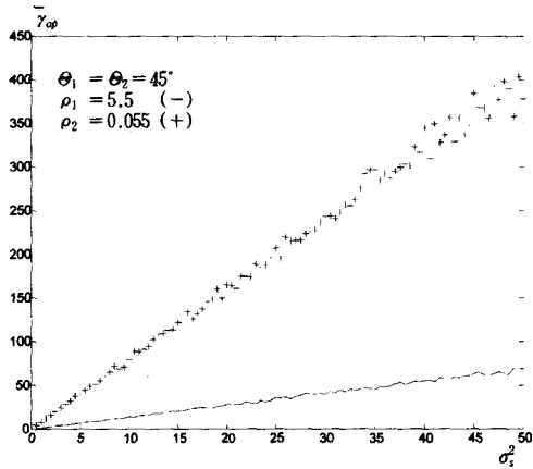
그림 6. 신호 대 간섭 잡음비와 퍼짐 관계
