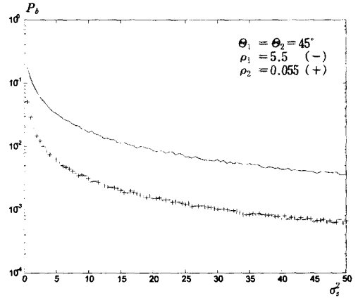
그림 7. 비트 오류 확률과 퍼짐 관계
