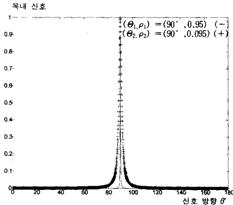
그림 3. 옥내 신호의 예
