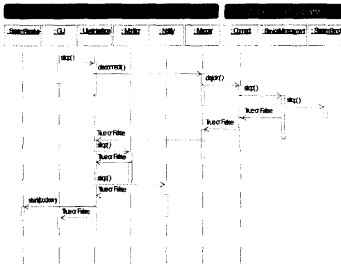
그림 22. 접속 해제 수행 절차의 시퀀스 다이어그램
