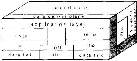
그림 4. Tenet 구조
