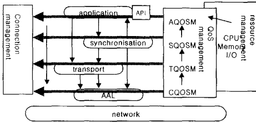
그림 5. MASI 구조
