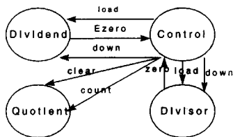
그림 1. 블록그래프
