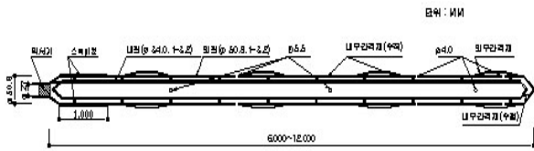
그림 7. TAS 주입볼트 구조도
