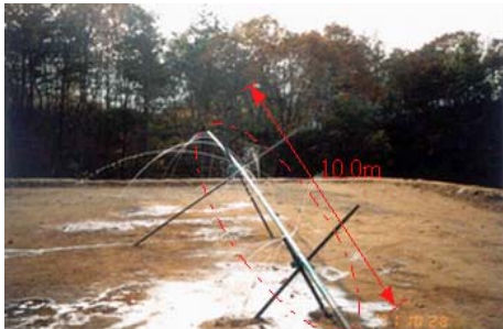
사진 8. TAS주입볼트의 약액 분출
