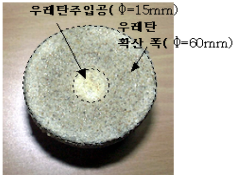
사진 3. 모래시료속에 주입된 우레탄 약액 2차 발포
