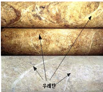
사진 13. 코어 샘플 상태
