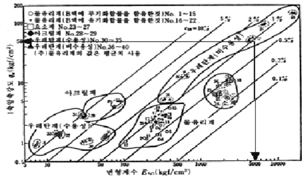
그림 2. 표준사고결토의 입출압축강도와 변형계수
