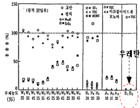
그림 3. 각 고결토의 용출성분 비교
