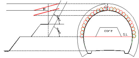
그림 4. 시공 각도
