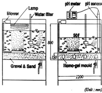
(a) 순용수조 (b) 시험수조 그림 8. 어독성 시험장치
