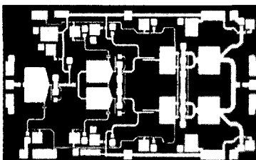
그림 7. 구동 전력 증폭기의 MMIC chip
