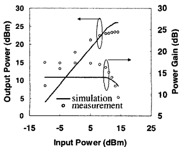
그림 8. 구동 전력 증폭단의 전력 특성
