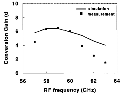
그림 9. 혼합기의 변환 이득
