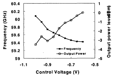
그림 4. Oscillation frequency와 power의 관계
