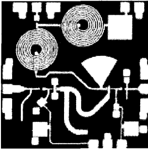
그림 11. 혼합기의 MMIC chip
