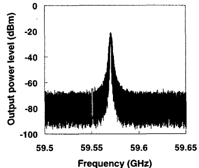
그림 5. Unmodified Spectrum
