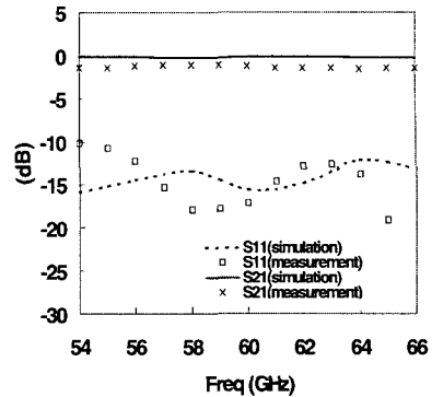
그림 14. Finline 변환 구조의 손실 특성
