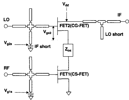
그림 10. cascode 혼합기의 구조도
