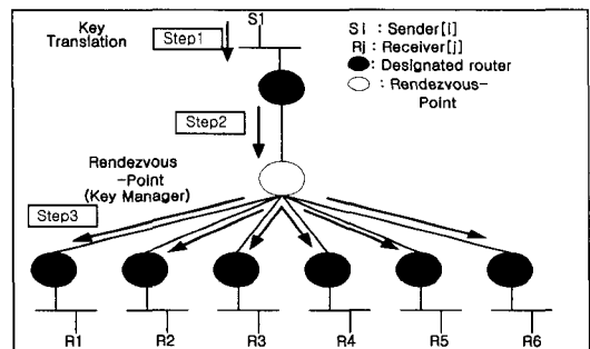
[그림 1] PIM-SM 그룹 키 관리 구조
