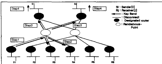
[그림 6] 수신자 탈퇴 과정 [Fig. 6] Receiver Leave Phase
