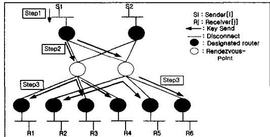
[그림 4] 송신자 탈퇴과정 [Fig. 4] Sender Leave Phase
