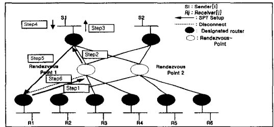
[그림 7] SPT 경로 설정 [Fig. 7] SPT Path Selection
