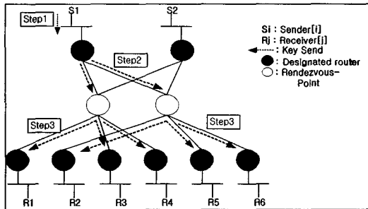
[그림 8] 데이터 전송 과정 [Fig. 8] Data Transmission Phase
