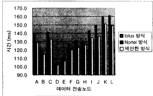
그림 12] 데이터 전송 평균 시간
