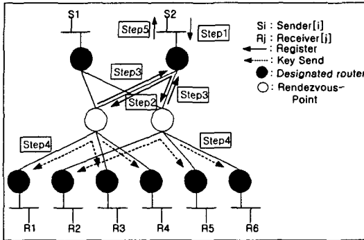
그림 3 송신자 등록 과정
