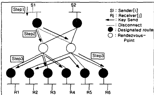
그림 4 송신자 탈퇴과정
