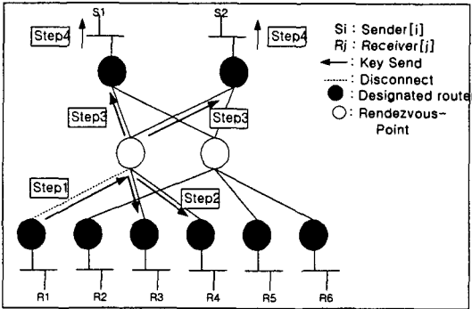
그림 6 수신자 탈퇴 과정
