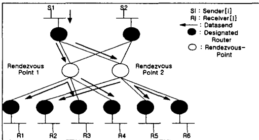
그림 11 제안된 방식의 데이터 전송과정
