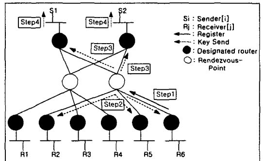
그림 5 수신자 등록과정
