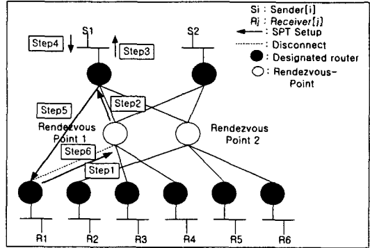
그림 7 최短路徑 設定
