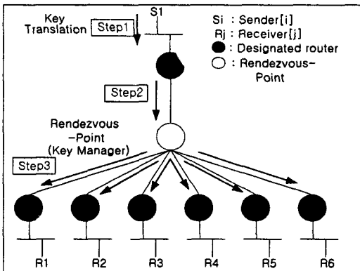
그림 1 PIM-SM 그룹 키 관리 구조
