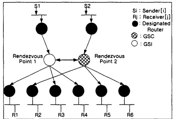
그림 9 Iolus 방식의 데이터 전송과정
