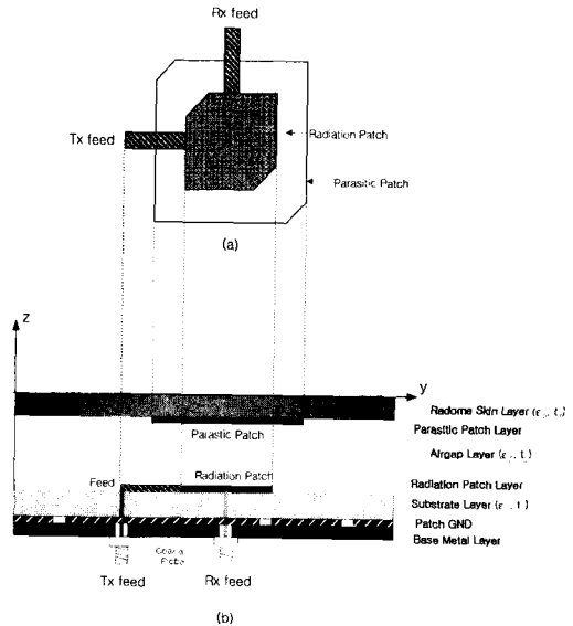
그림 1. 단일 방사소자의 구조 (a)윗면 (b)단면
