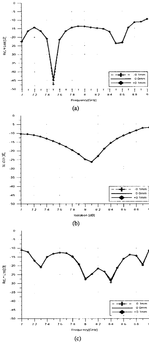
그림 7. 층간 어라인 오차에 따른 시뮬레이션 비교 결과 (a) 수신 port 반사손실 (b) 송/수신 간의 격리도 (c) 송신 port 반사손실
