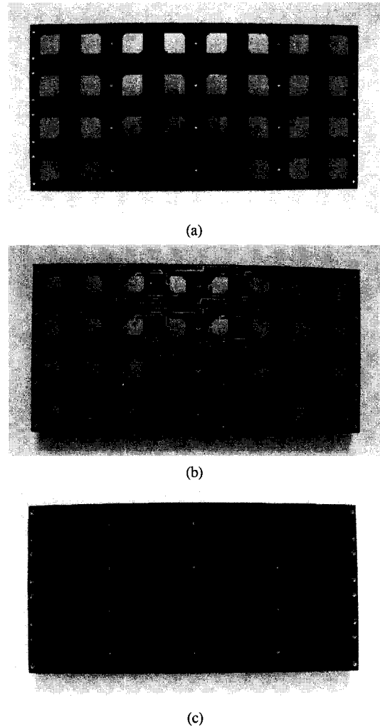
그림 8. 실제 제작된 송/수신 겸용 배열 안테나 (a) Parasitic patch layer 뒷면 (b) Radiation patch layer 앞면 (c) 조립된 송/수신 겸용 배열 안테나의 앞면
