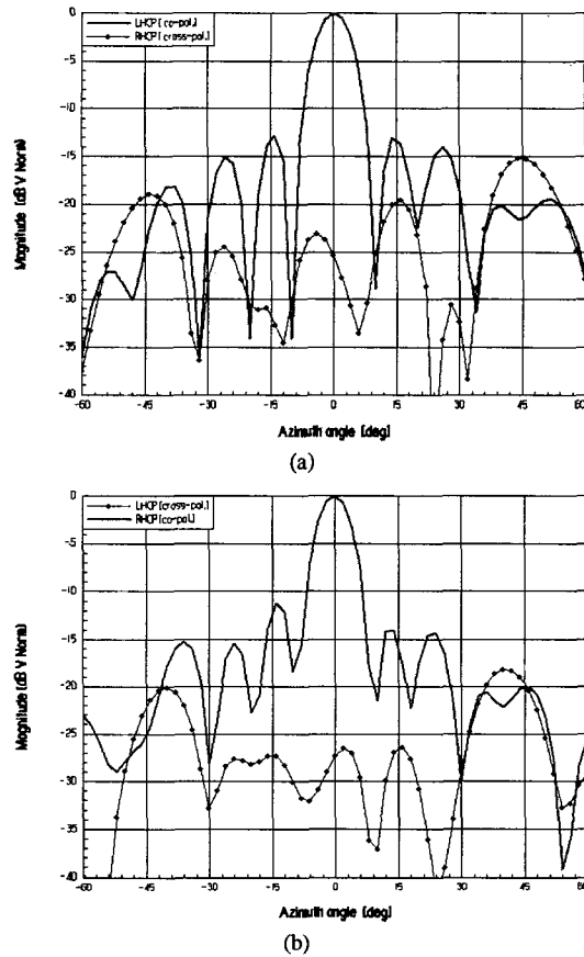
그림 6. 8x1 배열 안테나의 방위각 방향 방사패턴 시뮬레이션 결과 (a) f_{c\_rx}=7.5GHz (b) f_{c\_tx}=8.15GHz
