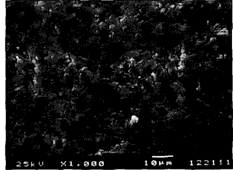
Fig. 2. 1군(2분, 8°C)의 주사전자현미경 사진( \times 1,000 )
