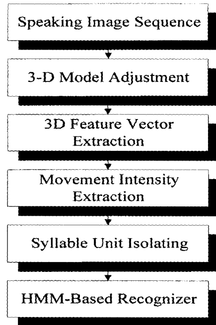
그림 1. 전체 영상처리 과정 Fig. 1 Image Processing
