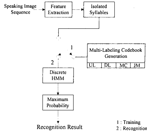
그림 6. 이산HMM 인식기 Fig. 6 Discrete HMM Recognizer
