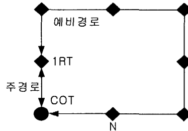
그림 5. 격자모형(성형망)
