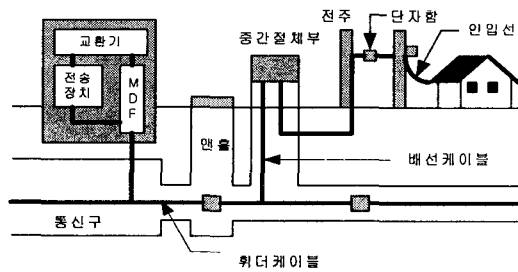
그림 1. 가입자망의 구성
