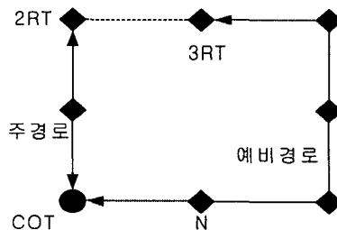
그림 6. 격자모형(링형망)
