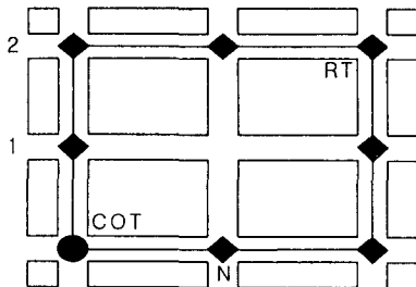
그림 4. 격자모형(N=7)
