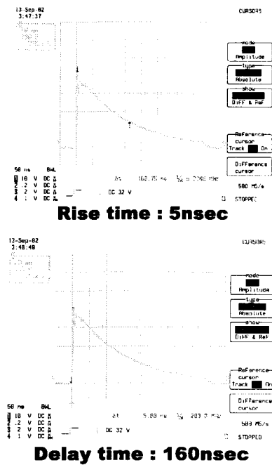
그림 6. HBM ESD tester의 rise 및 delay time Fig. 6 rise and delay time of waveform generated from HBM ESD tester
