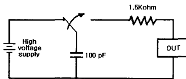
그림 1. HBM (Human Body Model) Fig. 1 HBM (Human Body Model)
