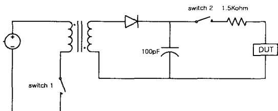
그림 4. 고전압 부분의 회로도 Fig. 4 Schematic of high voltage part
