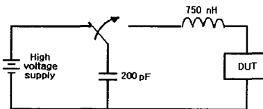
그림 2. MM (Machine Model) Fig. 2 MM (Machine Model)
