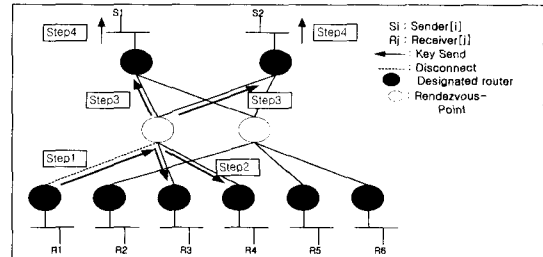
(그림 6) 수신자 탈퇴 과정
