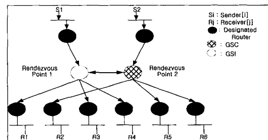
(그림 9) Iolus 방식의 데이터 전송과정
