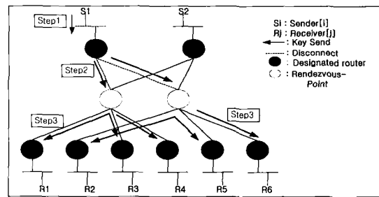
(그림 4) 송신자 탈퇴과정
