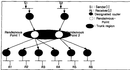
(그림 10) Nortel 방식의 데이터 전송과정
