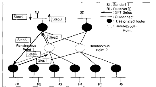
(그림 7) 최소거리경로 설정
