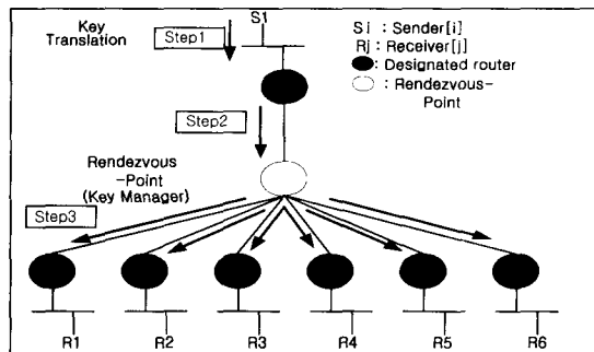
(그림 1) PIM-SM 그룹 키 관리 구조
