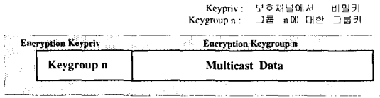
(그림 2) 암호화된 데이터 형식
