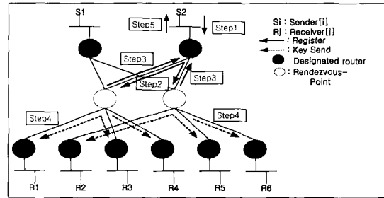
(그림 3) 송신자 등록 과정
