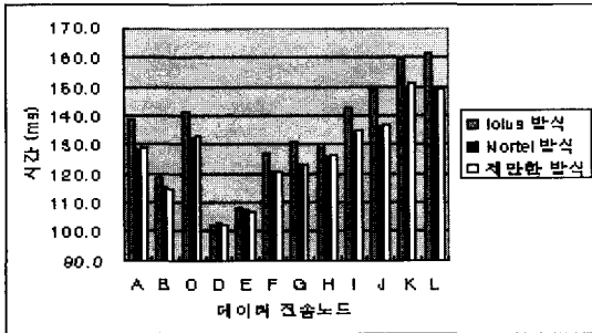
(그림 12) 데이터 전송 평균 시간
