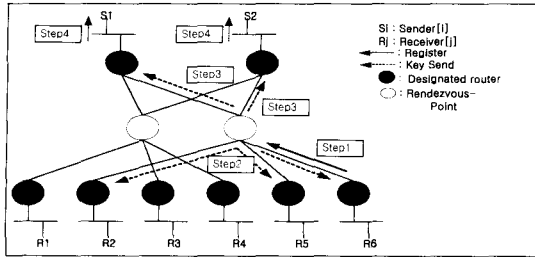
(그림 5) 수신자 등록과정
