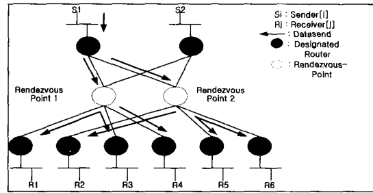
(그림 11) 제안된 방식의 데이터 전송과정
