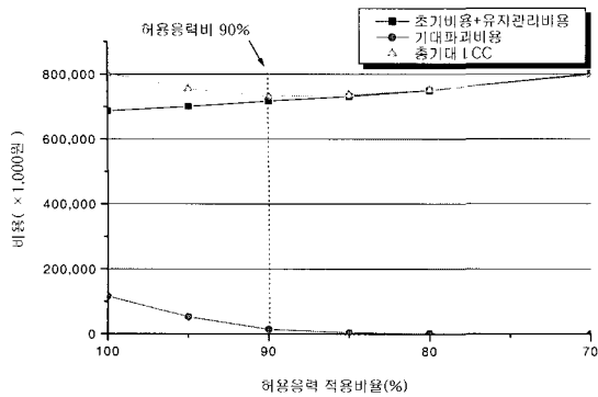
그림 6 허용응력 변화에 따른 주형의 총기대 LCC
