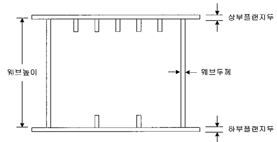
그림 2 주형의 설계변수
