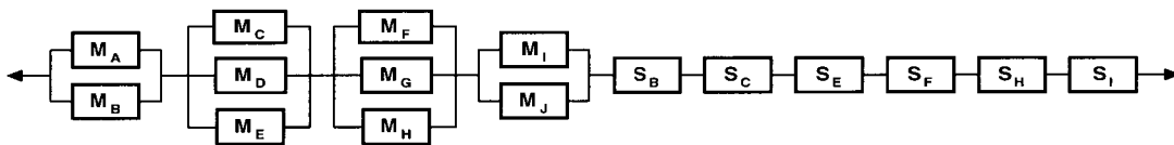
(b) 직·병렬시스템 모델
