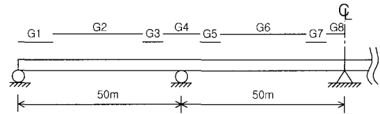
그림 5 종방향 단면그룹
