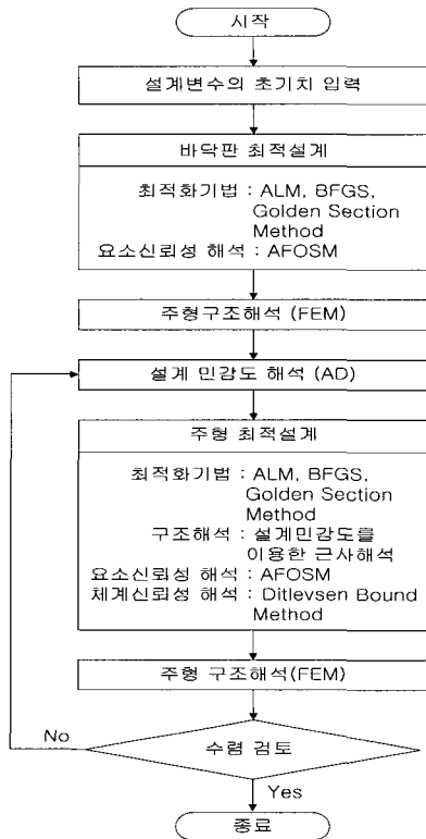
그림 4 강상자형교의 LCC 최적설계 알고리즘
