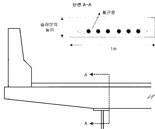
그림 1 바닥판의 설계변수
