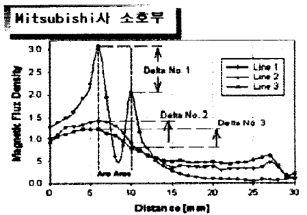
(a) 일본 M사 소호부의 구동자계
