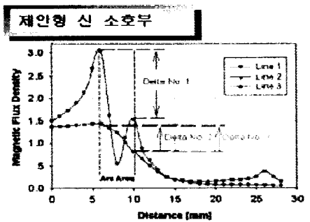
(b) 신소호부의 구동자계
