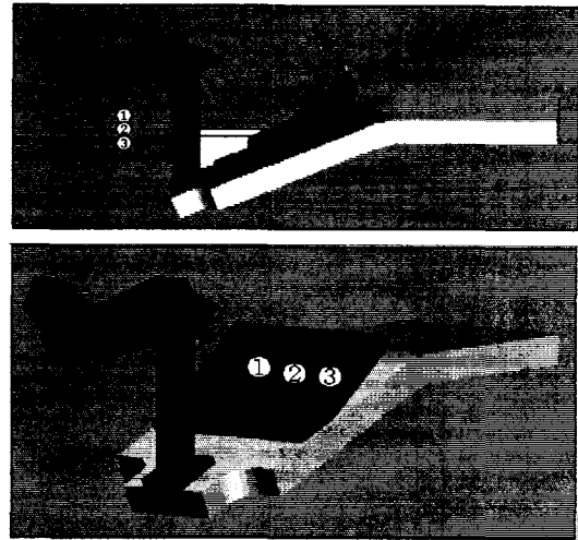
그림 1. 차단성능 평가를 위한 자계해석 기준선 Fig. 1. Analytic lines of magnetic flux for the estimation of the interrupting capability
