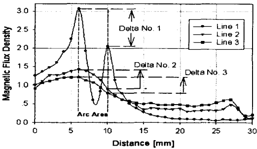
(d) 일본 M사 MCCB
