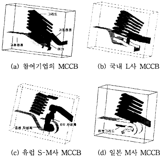
그림 3. 자계해석을 위한 차단기 소호부 형상 Fig. 3. Shapes of the contact systems for magnetic analysis
