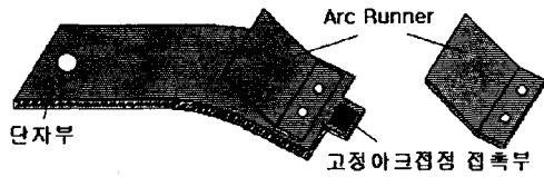
그림 5. 기준 고정아크접점 및 아크런너 Fig. 5. Basic stationary arc contact & runner
