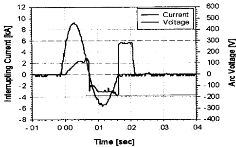
(f) 국내 L사 소호부
