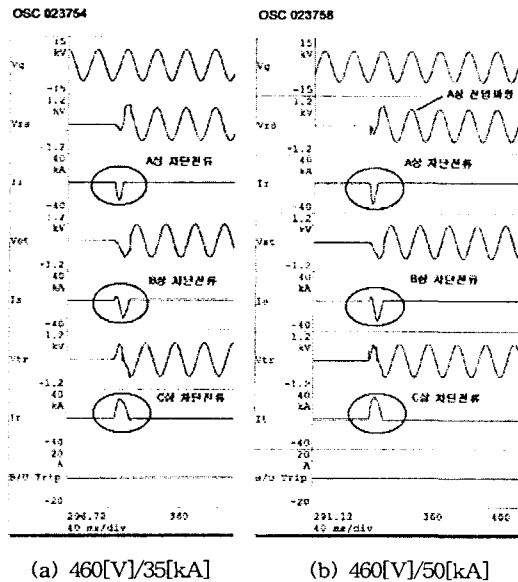
그림 11. 460[V]/35(kA)/50(kA) 대전력 차단시험 결과 Fig. 11. Results of current interrupting test under 460[V]/35(kA)/50(kA)
