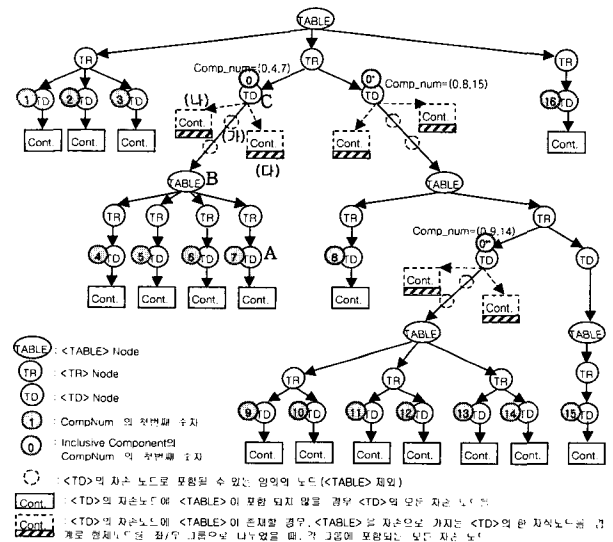
(그림 7) (그림 4)의 HTML 예제의 구조적 태그 집합의 트리 모형
