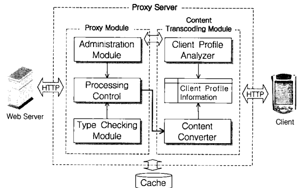
(그림 10) 웹 문서 변환기와 프락시 서버 모듈간의 연동 구성도
