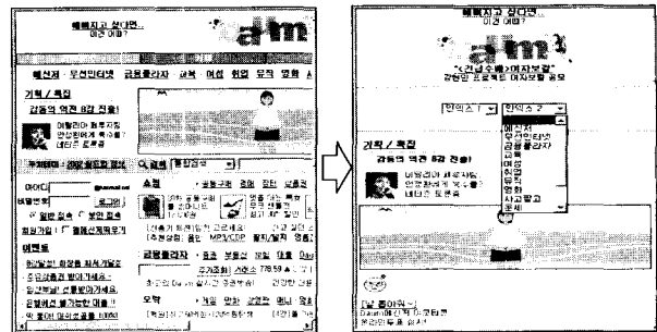
(그림 12) Daum 사이트를 변환한 결과(MAX_WIDTH = 400)
