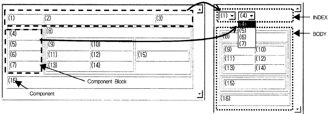
(그림 2) 웹 문서 변환 기법의 주요 예제도(좌 : 변환 전, 우 : 변환 후)
