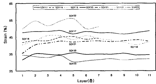
그림 9. SDY 75d/36f의 Maker별 layer 간의 절단신도
