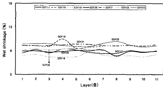
그림 12. SDY 75d/36f의 Maker별 layer 간 습열 수축률의 변화 (Hank법)
