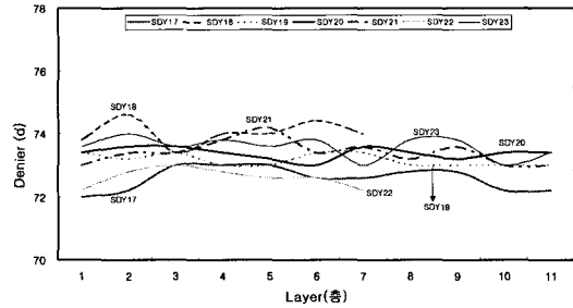
그림 5. SDY 75d/36f의 Maker별 layer 간의 섬도 변화
