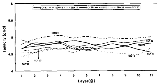
그림 8. SDY 75d/36f의 Maker별 layer 간의 절단강도
