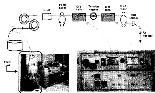
그림 1. Toray Fibre Thermal Analysis (FTA-500, Japan, Toray, ENG.)
