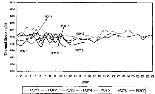
그림 14. POY(85d/72f)의 Maker별 Layer간 열응력 변화
