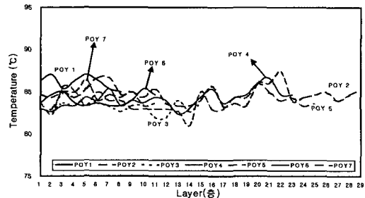
그림 15. POY(85d/72f)의 Maker별 최대 열응력 온도
