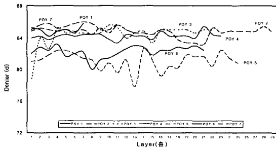
그림 3. POY 85d/72f의 Maker별 layer 간의 섬도 변화
