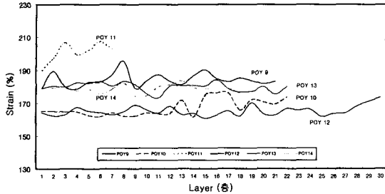
그림 7. POY 120d/36f의 Maker별 layer 간의 절단 신도
