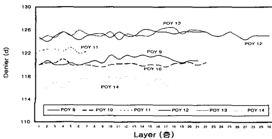
그림 4. POY 120d/36f의 Maker별 layer 간의 섬도 변화
