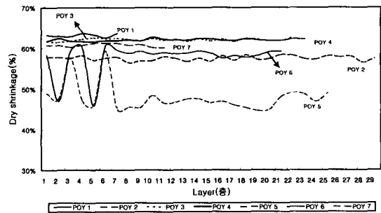
그림 10. POY 85d/72f의 Maker별 layer 건열 수축률의 변화 (hank 법)
