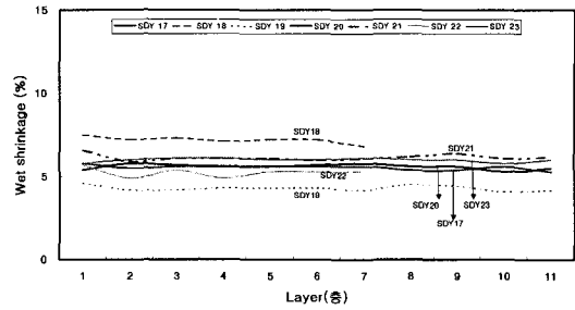
그림 13. SDY 75d/36f의 Maker별 layer 간 습열 수축률의 변화 (Toray 법)
