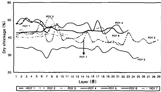
그림 11. POY 85d/72f의 Maker별 layer 건열 수축률의 변화 (Toray 법)
