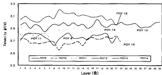
그림 6. POY 120d/36f의 Maker별 layer 간의 절단 강도
