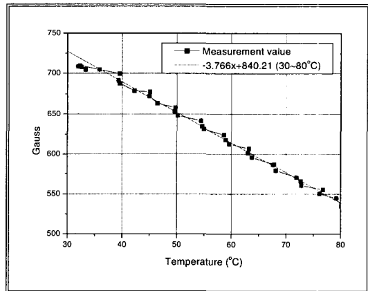
그림 3. 페라이트 영구자석 온도특성. Fig. 3. Temperature characteristics of permanent magnetic ferrite.
