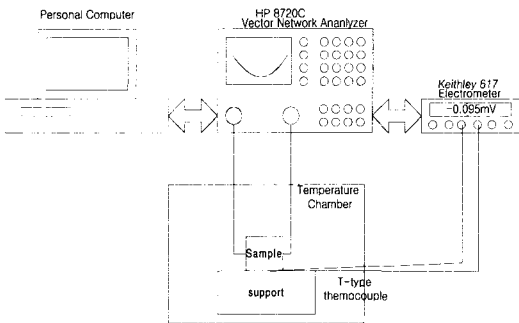
그림 2. 아이솔레이터 온도특성 측정시스템 구성. Fig. 2. Constitution for temperature characteristics measurement system of Isolator.
