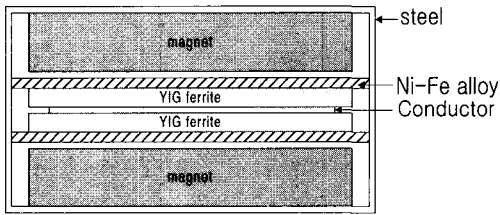
그림 1. 아이솔레이터 단면도. Fig. 1. Cross section of Isolator.
