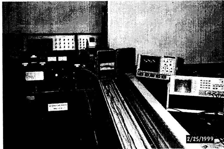
<그림 2> 스위칭 유도노이즈 측정 실험장치
